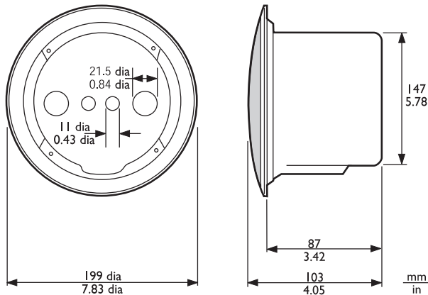
Kích thước của bộ Vòm Chống cháy LBC 3090/31 + LBC 3080/01 tính theo mm (in)
