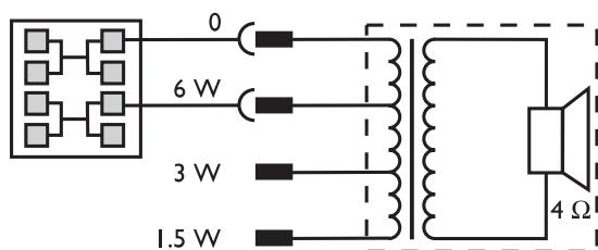
Sơ đồ nối mạch
